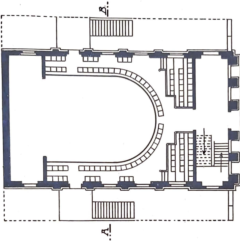
Salão de conferências: Planta da galeria
